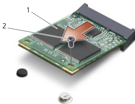
1 FCM カード 2 M2 x 3 mm 固定ネジ
