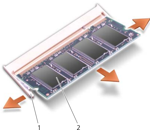
1 固定クリップ (2) 2 メモリモジュール (DIMM 1)
