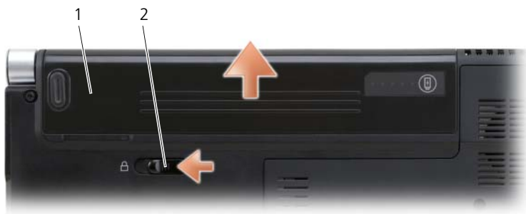
1 バッテリー 2 バッテリーリリーススラッチ
