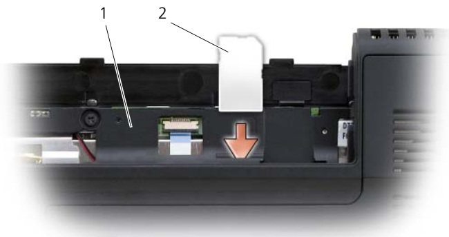
1 バッテリーバイ 2 SIM
